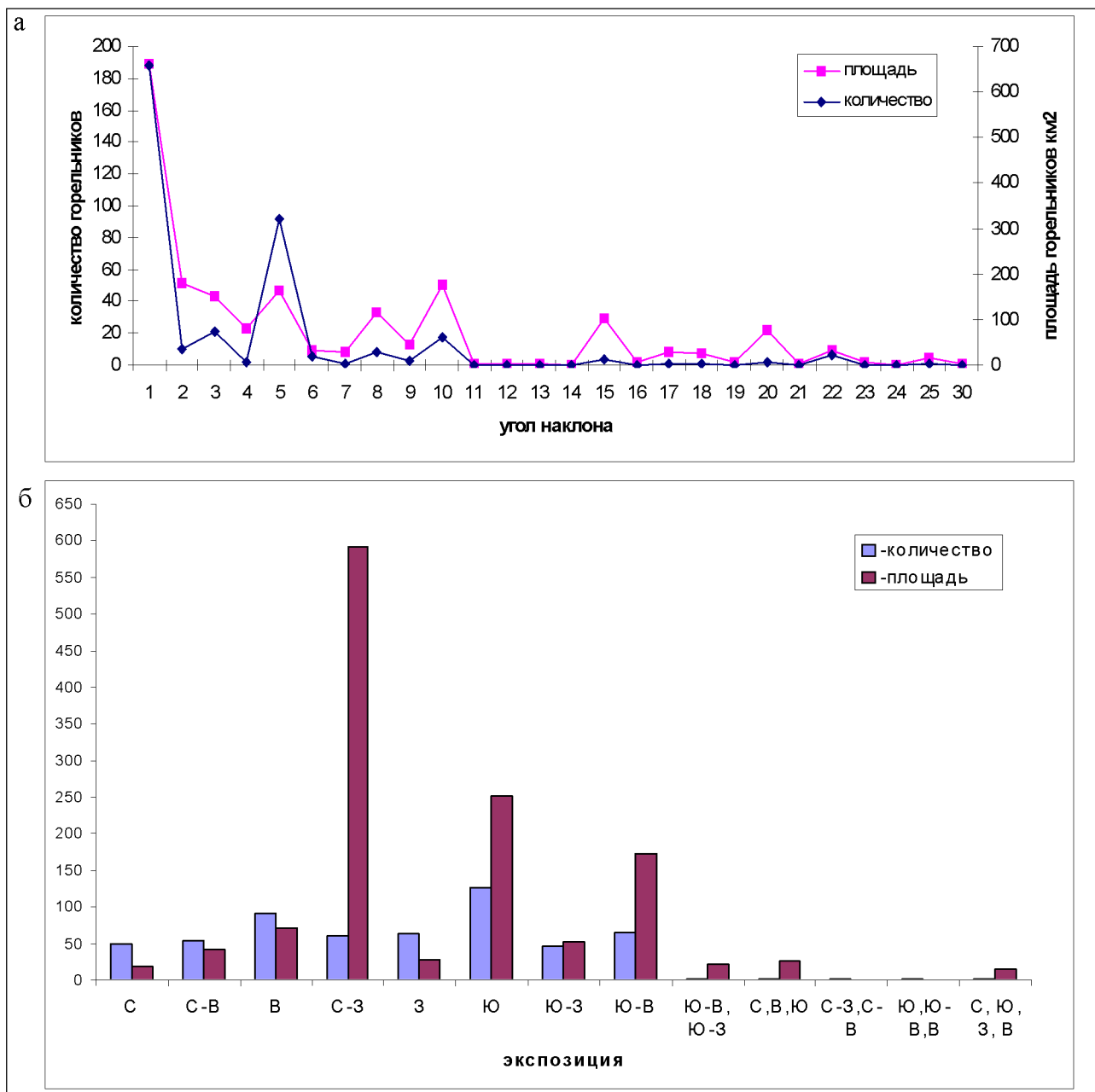
Рис. 2. Влияние на пожароопасность территории Еврейской автономной области геоморфологических характеристик: а) угла наклона б) экспозиции склона
