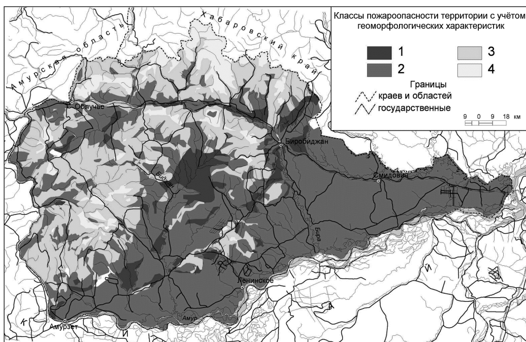
Рис. 3. Районирование территории Еврейской автономной области по пожароопасности с учётом геоморфологических особенностей
