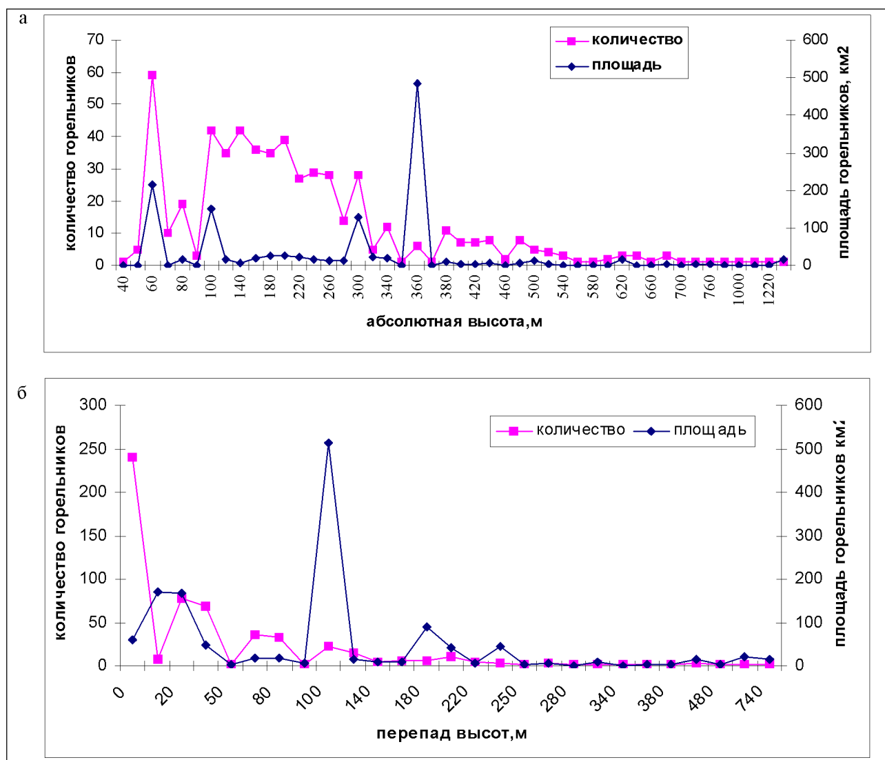
Рис. 1. Влияние геоморфологических показателей на численность и площадь горельников на территории Еврейской автономной области: а) абсолютная высота; б) перепад высот
